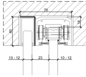
Typ C: Einbau
