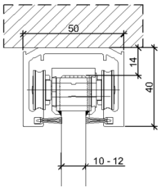
Typ A: Deckenmontage
