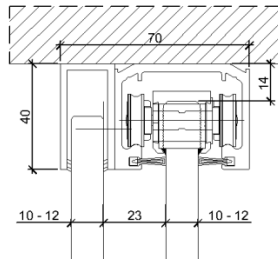
Typ B: Deckenmontage mit Fixteil
