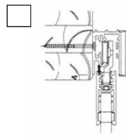
Typ B: Wandmontage
