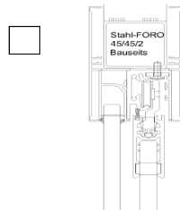
Typ F: Deckenmontage mit Fixteil
