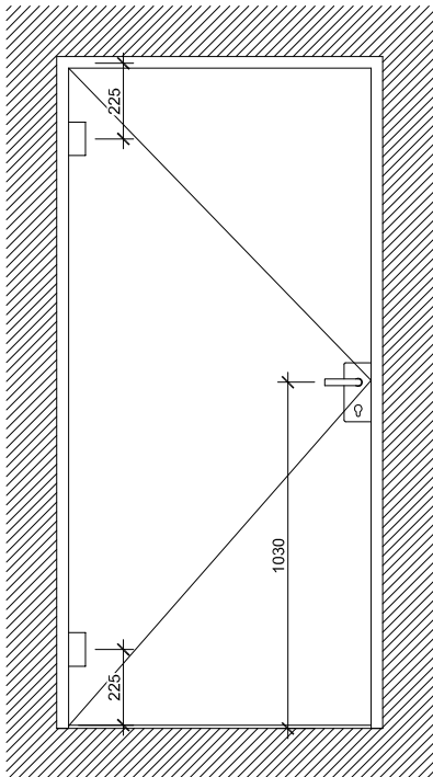
Türe DIN Rechts
